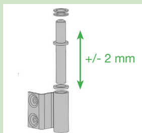
Paumelle réglable en hauteur
